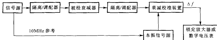
图1 衰减器检定系统方框图
