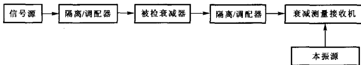
图 3 衰减器检定系统方框图
